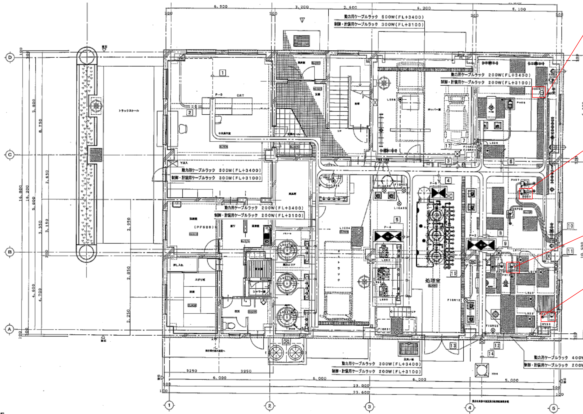
1 階平面図 1/100
