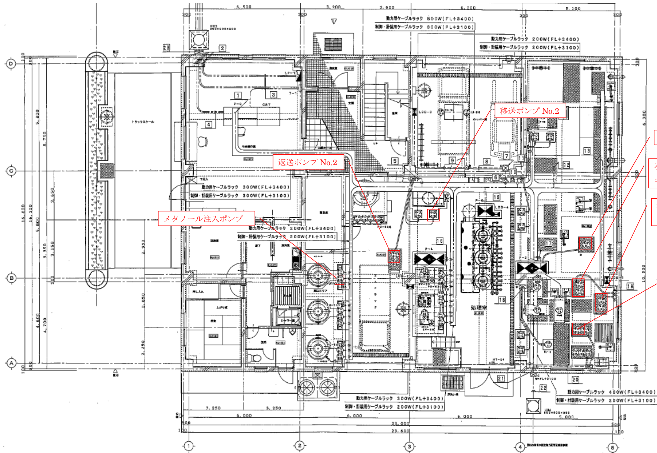
1階平面図 301/40
