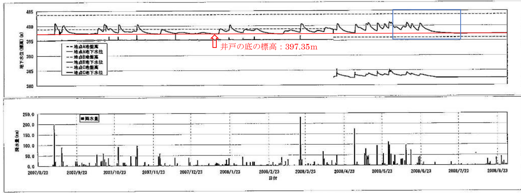
図 4.6. 1-10 (1) 観測井の浅層地下水の水位変化及び降水量の経時変動
